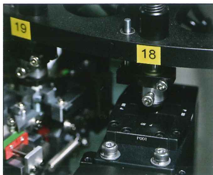
3D5S 視覺檢查系統 3D5S Color CCD inspection system
